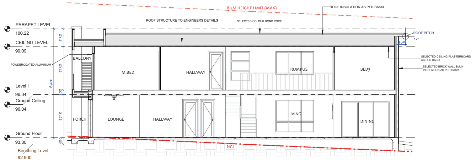
2 LONGITUDINAL SECTION 1 : 100
