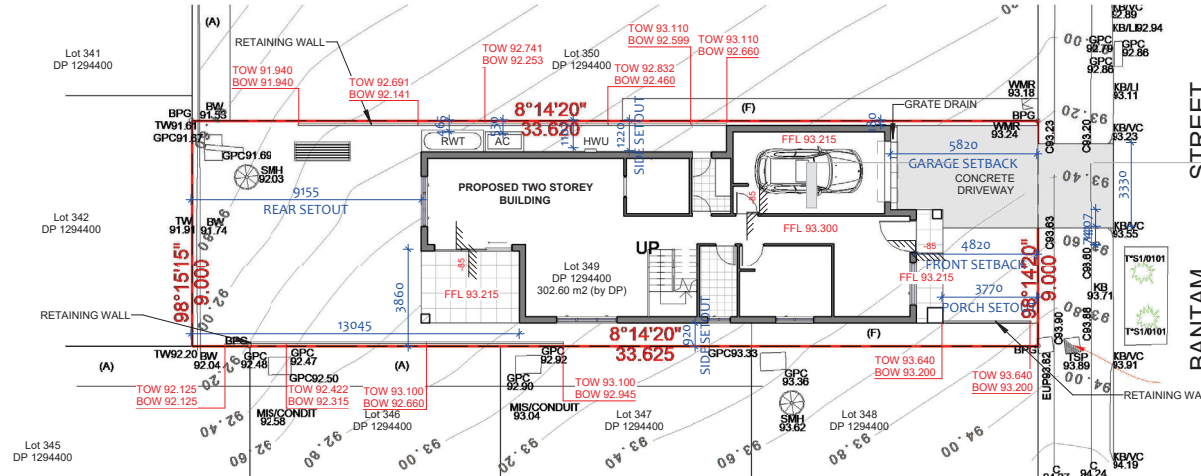
1 SITE PLAN 1 : 200
