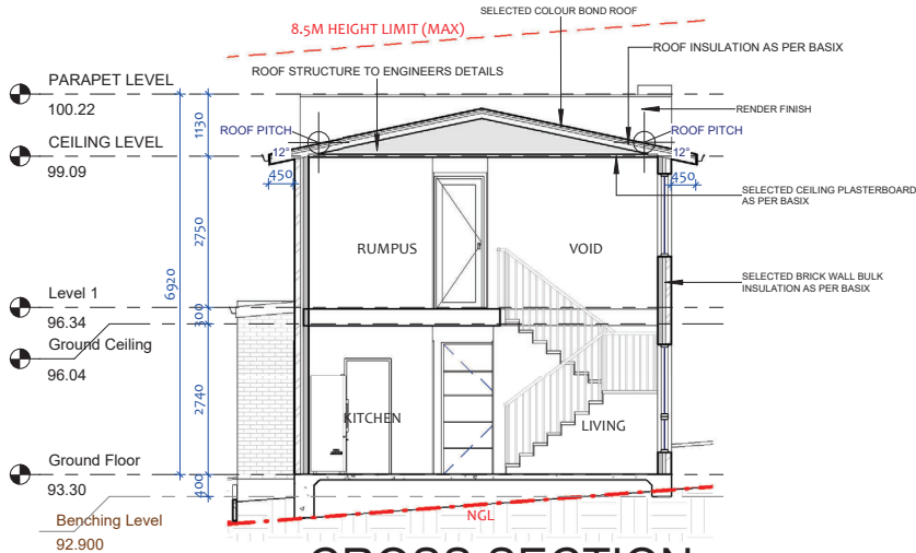
1 CROSS SECTION 1 : 100
