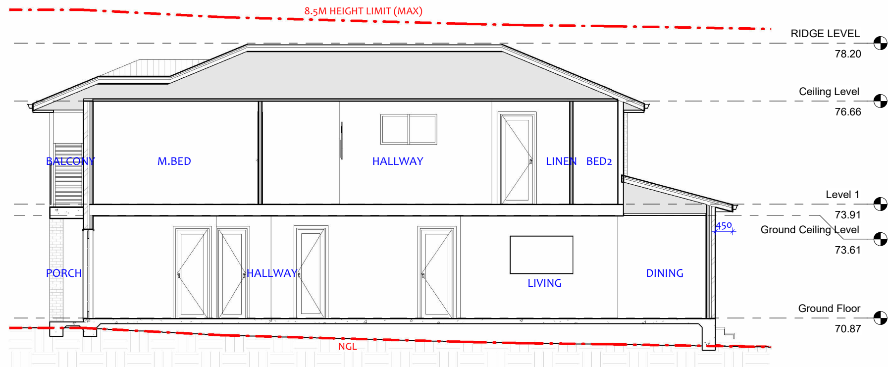
1 LONGITUDINAL SECTION 1 : 100
