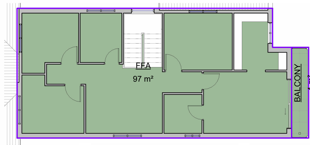
2 Level 1 1 : 100
