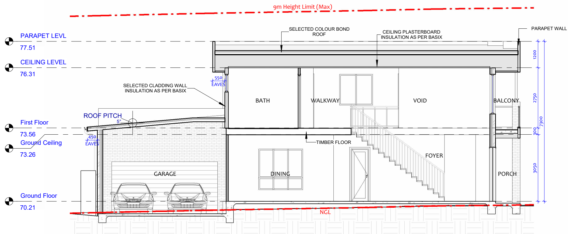
2 LONGITUDINAL SECTION 1 : 100
