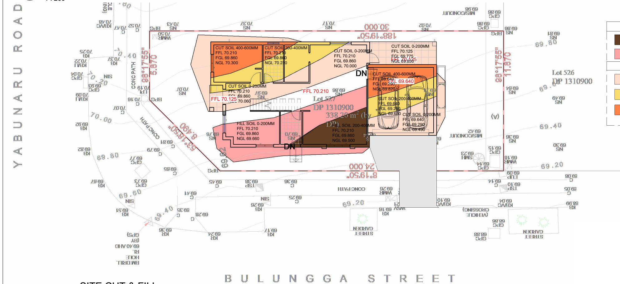
SITE CUT & FILL
