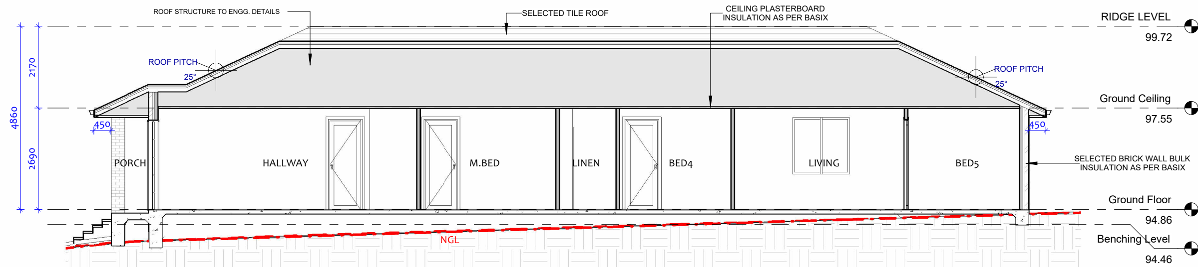
1 LONGITUDINAL SECTION 1 : 100
