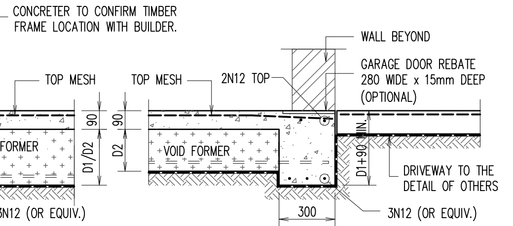
GARAGE EDGE BEAM – 'EB3'
