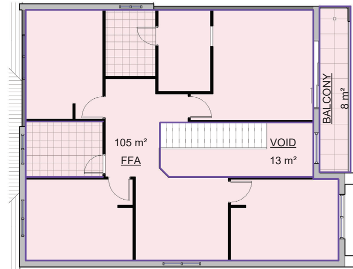
2 Level 1 1 : 100
