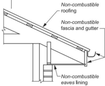
(d) Eaves construction
