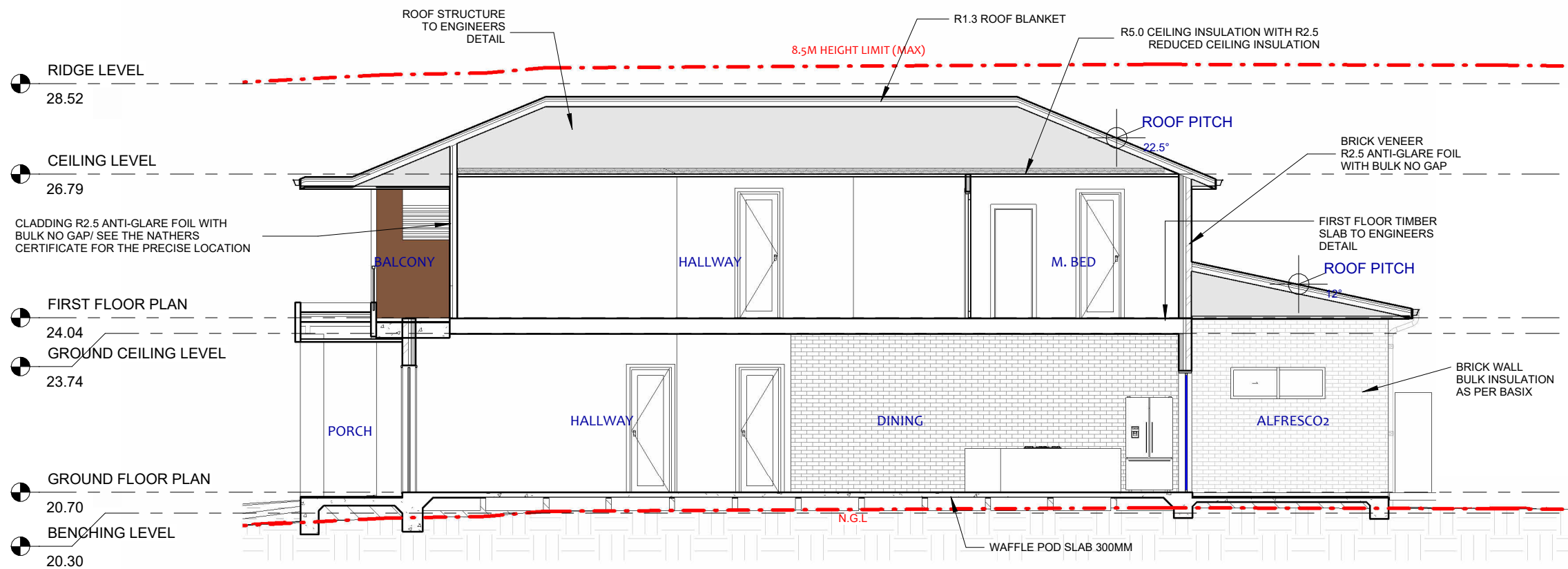
2 LONGITUDINAL SECTION 1 : 100
