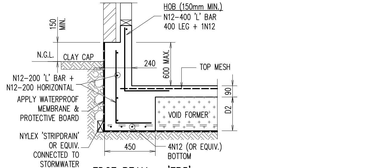
EDGE BEAM – 'EB5'
