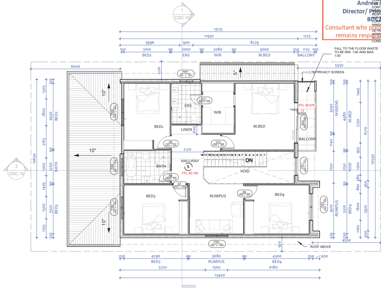
1 Level 1 1 : 100
