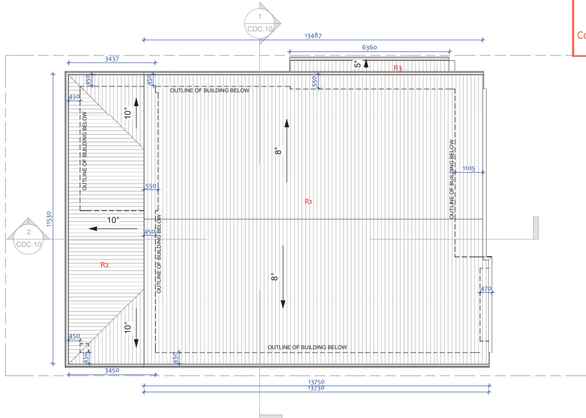
1 ROOF PLAN 1 : 100
