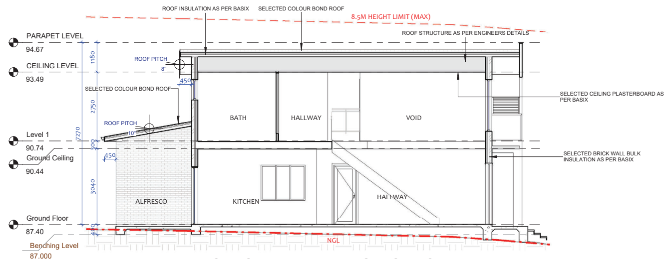
2 LONGITUDINAL SECTION 1 : 100
