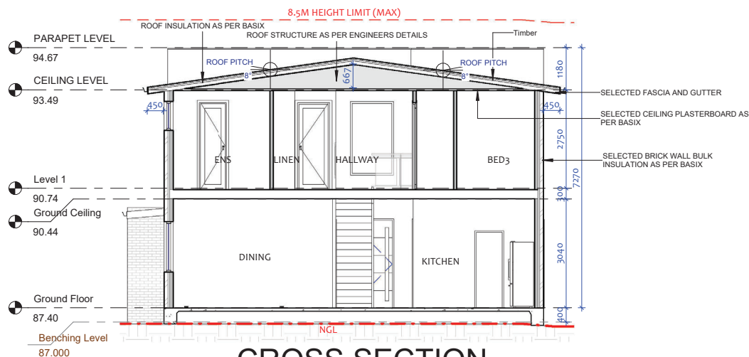
1 CROSS SECTION 1 : 100
