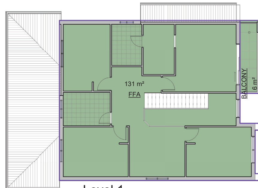
2 Level 1 1 : 100
