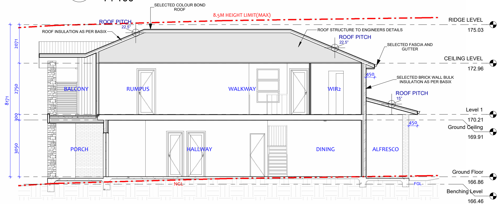
1 LONGITUDINAL SECTION 1 : 100
