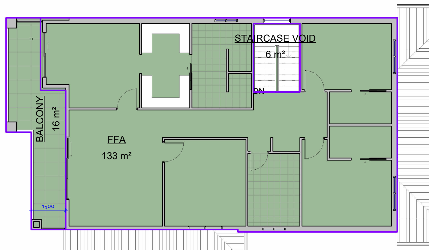
2 Level 1 1 : 100
