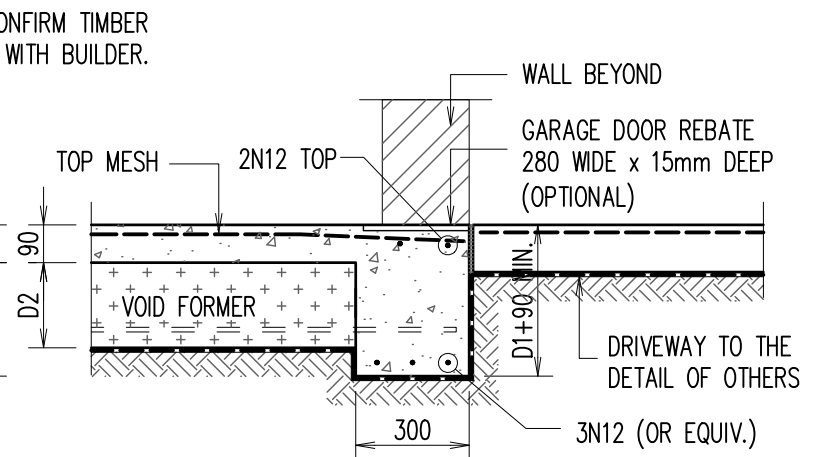
GARAGE EDGE BEAM – 'EB3'
