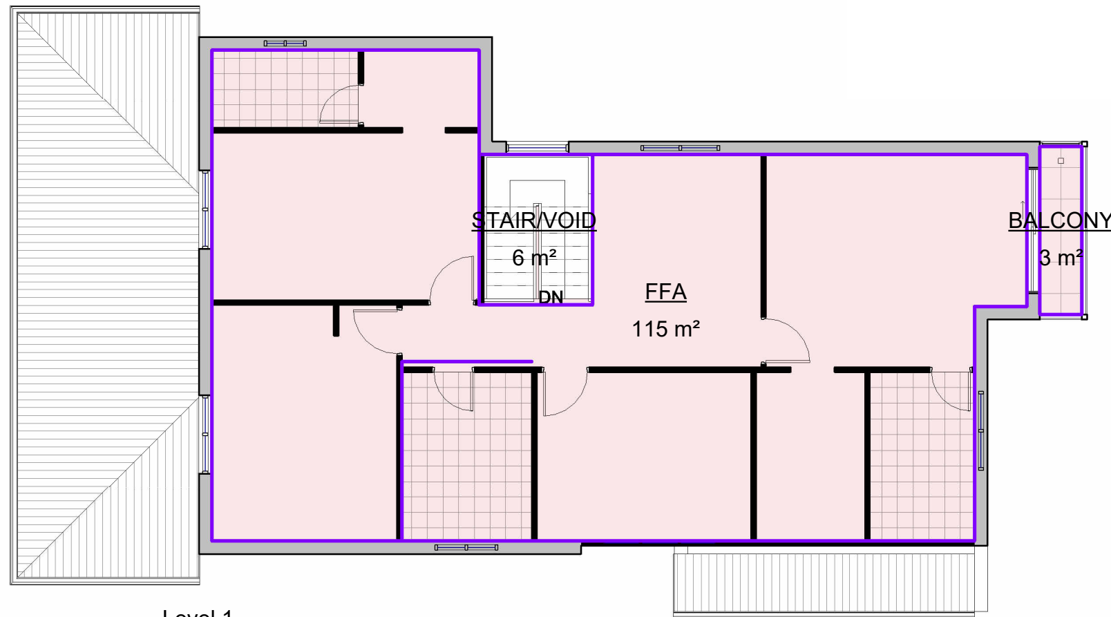
2 Level 1 1 : 100
