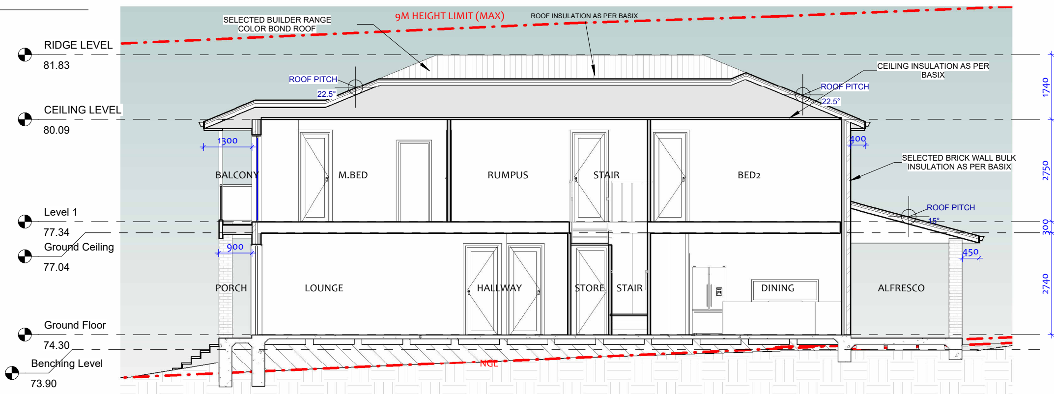
LONGITUDINAL SECTION
