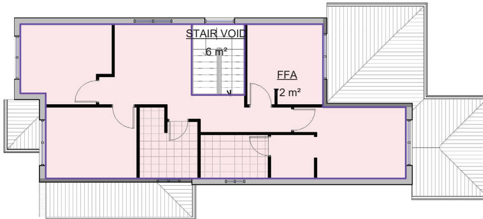
2 Level 1 1 : 100
