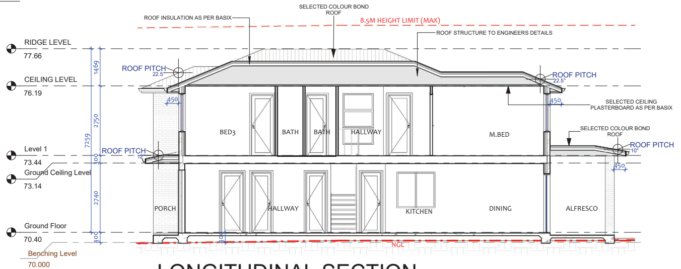
2 LONGITUDINAL SECTION 1 : 100
