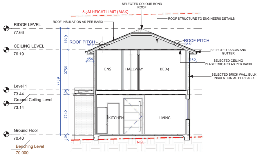
1 CROSS SECTION 1 : 100
