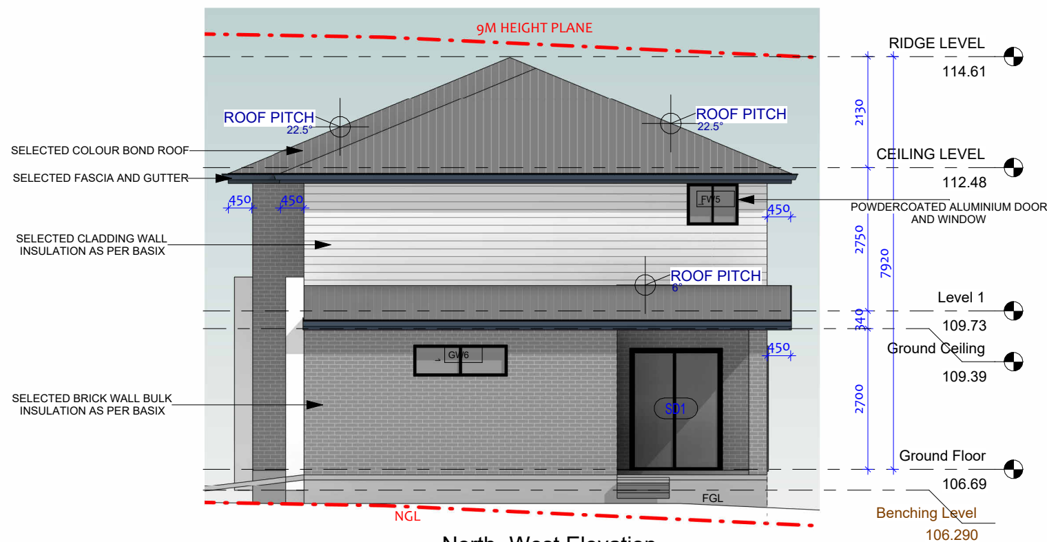
2 1 : 100
