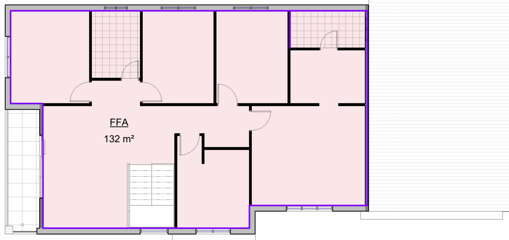
2 Level 1 1 : 100
