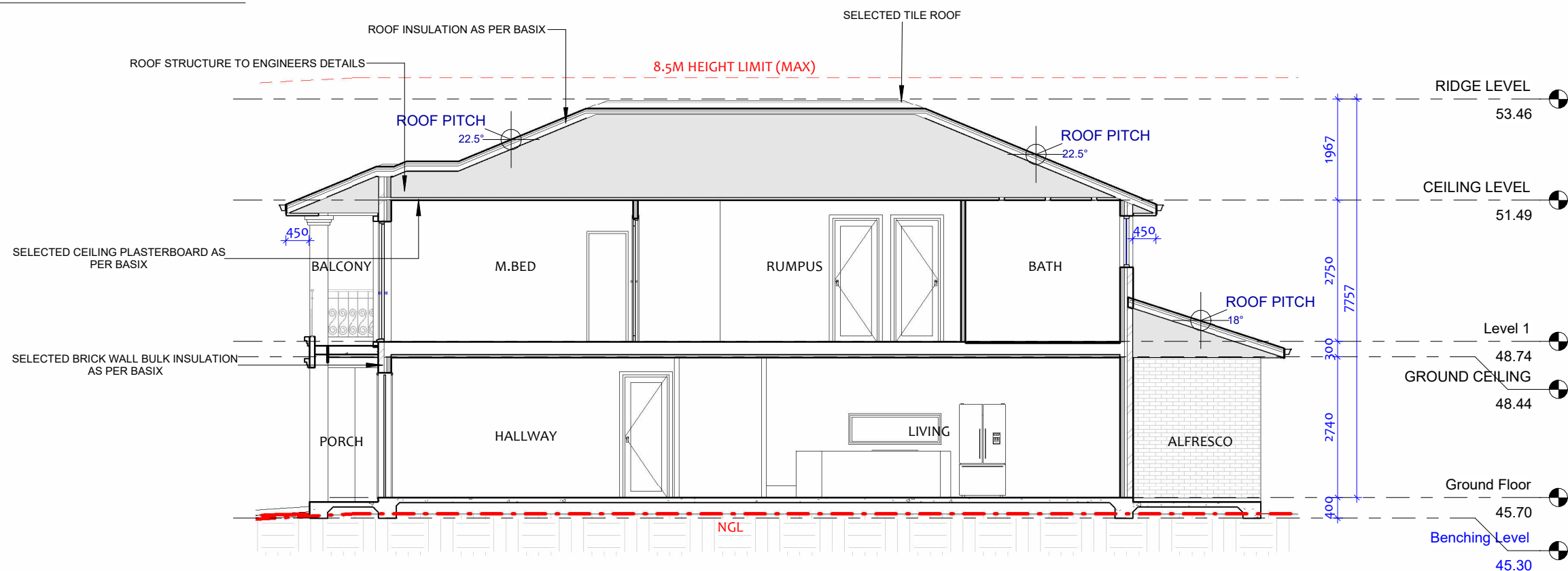
2 LONGITUDINAL SECTION 1 : 100
