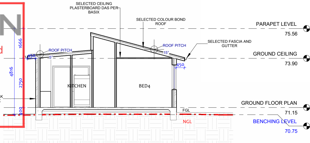
CROSS SECTION 1 1 : 100
