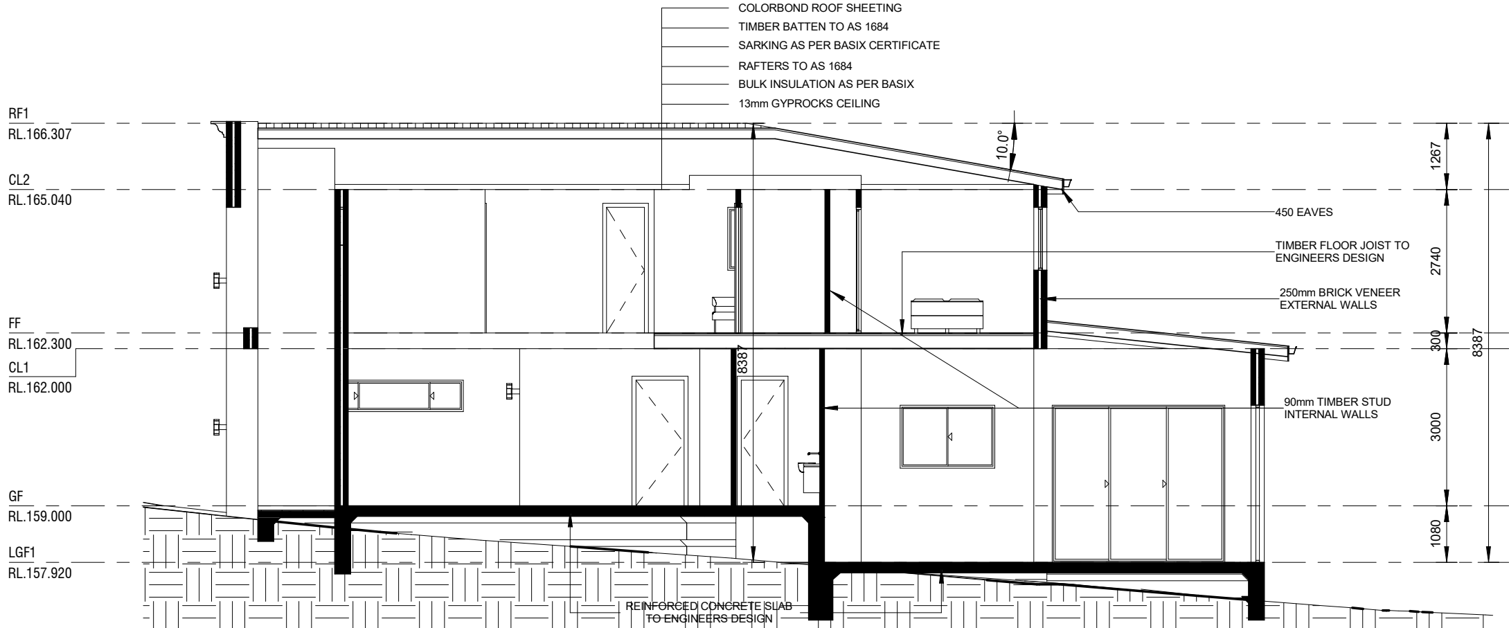
2 A05 SECTION - DW1 1 : 100
