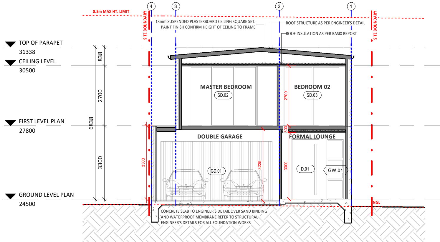
1 SECTION AA' 1 : 100
