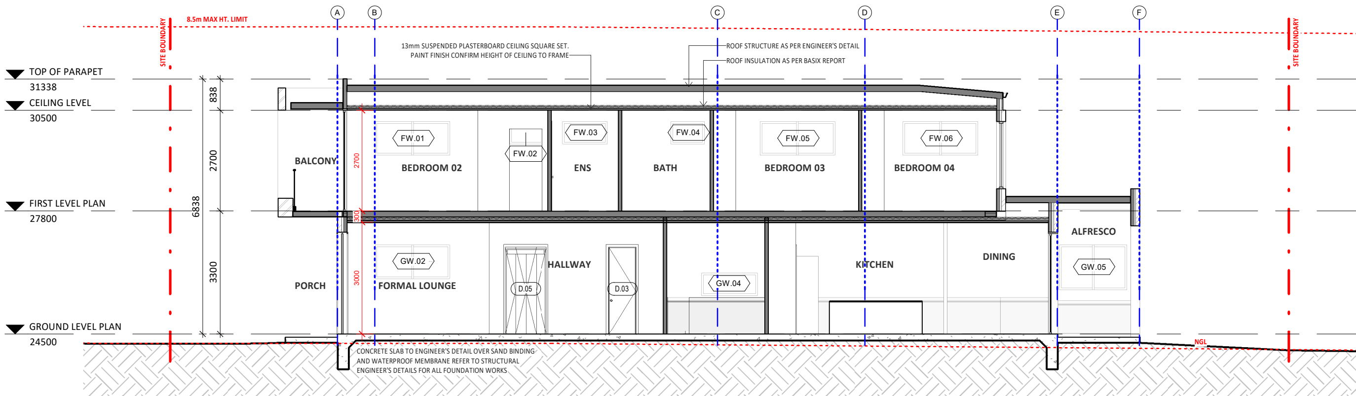
2 SECTION BB' 1 : 100
