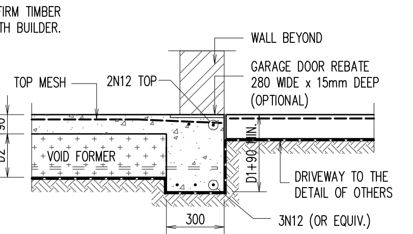
GARAGE EDGE BEAM – 'EB3'
