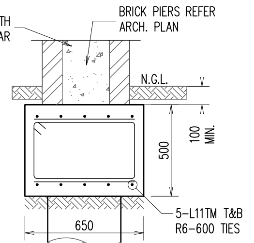
GARAGE EDGE BEAM – 'EB3'
