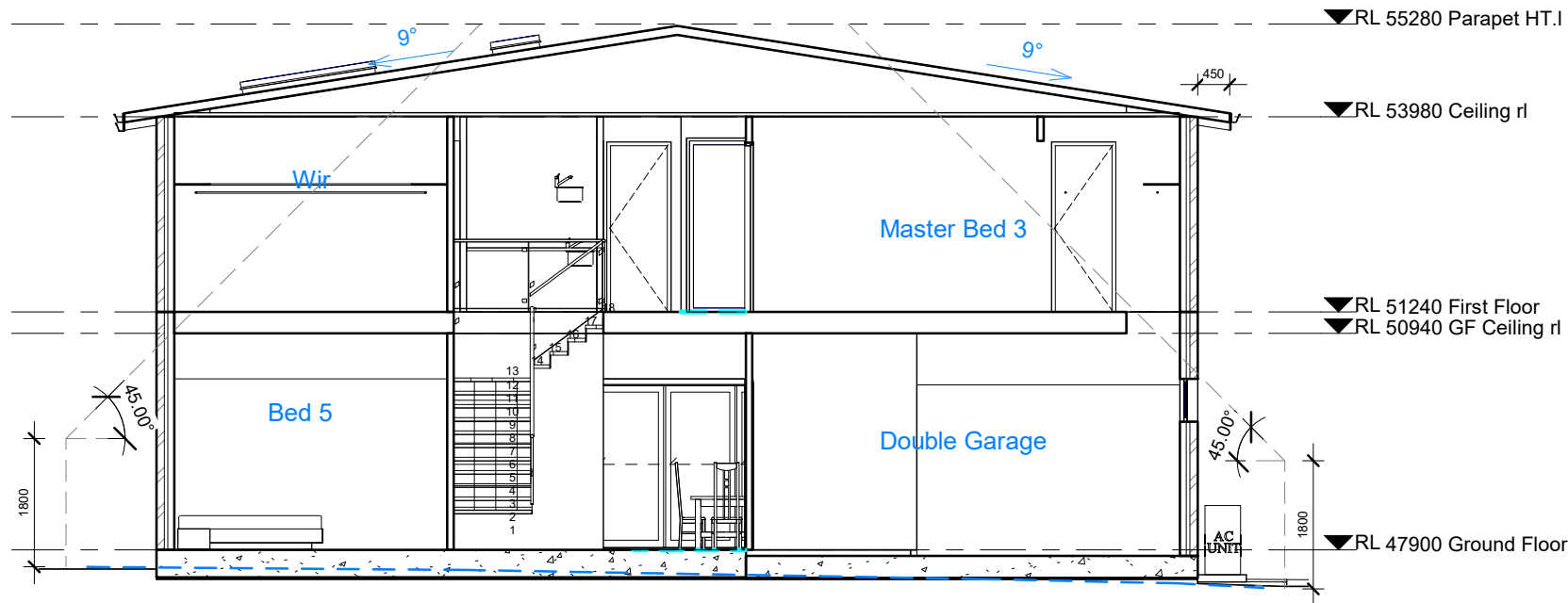
Section 1 1 : 100
