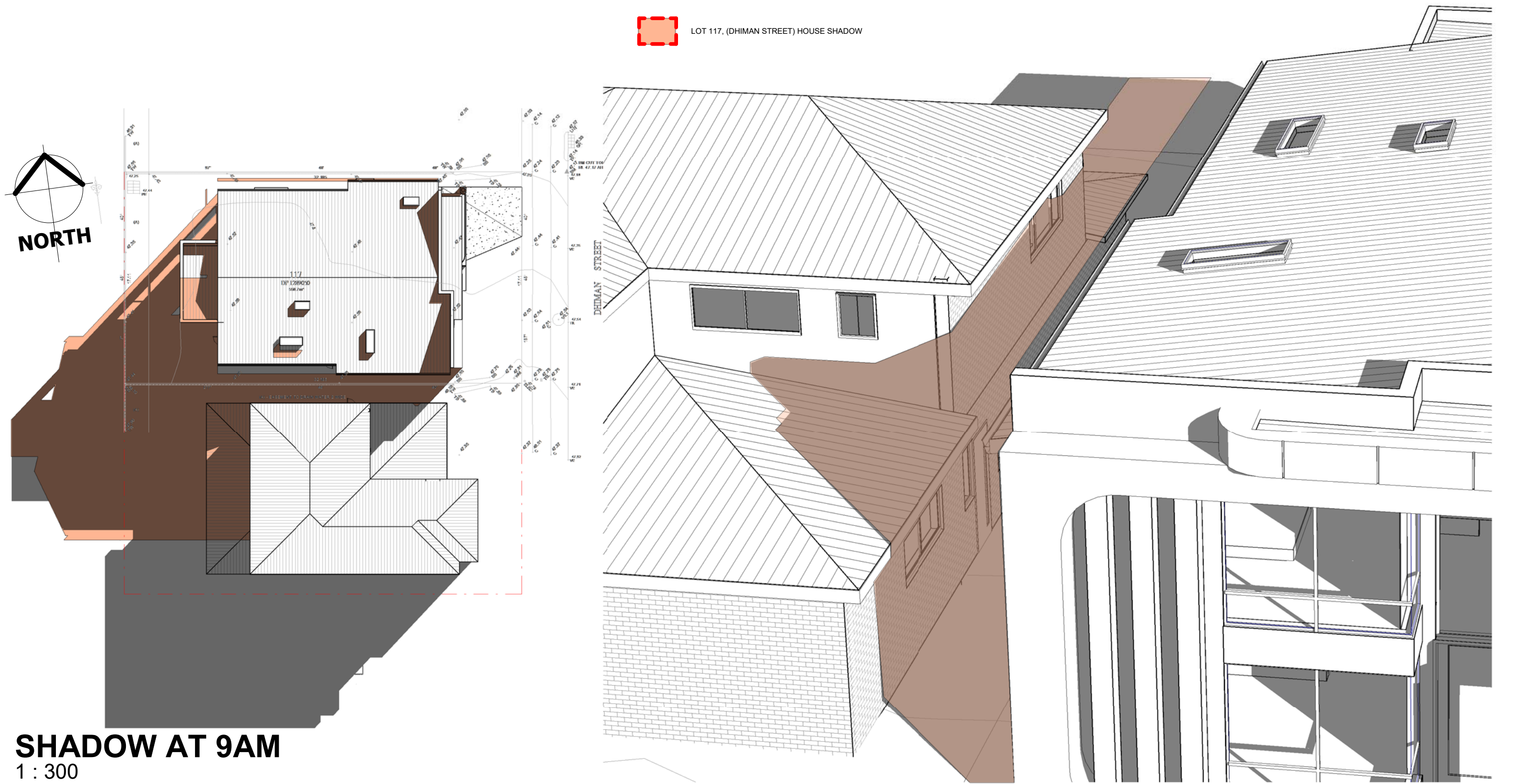
Shadow @ 9AM
