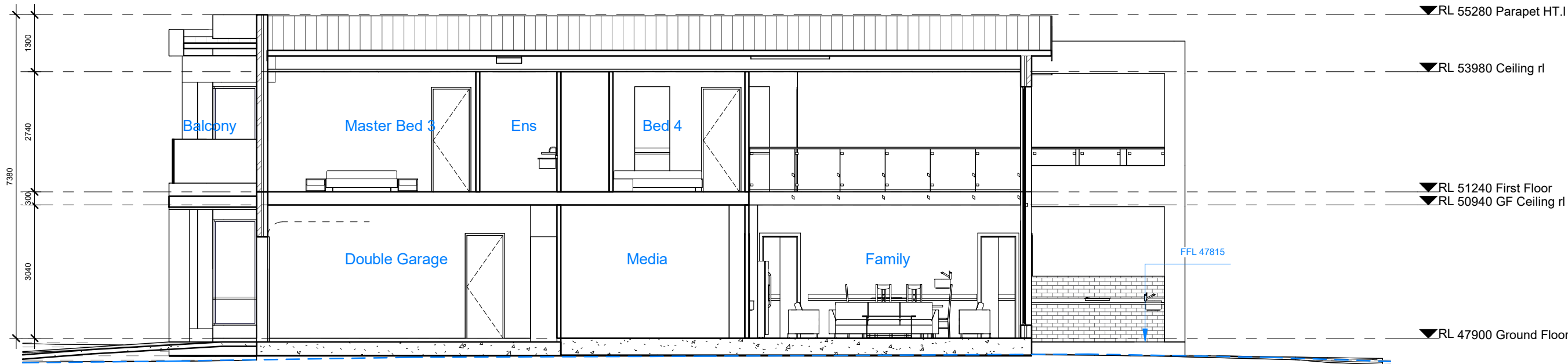
Section 2 1 : 100
