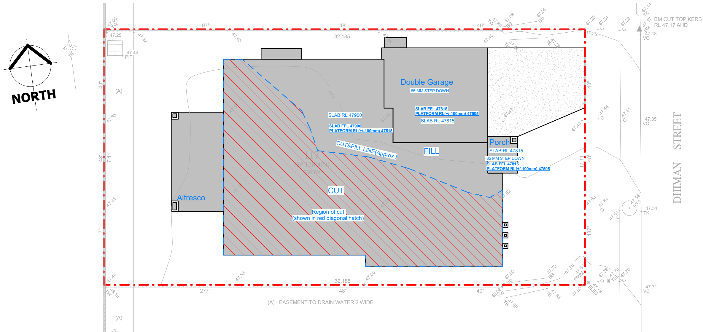
Cut & Fill Plan 1 : 150
