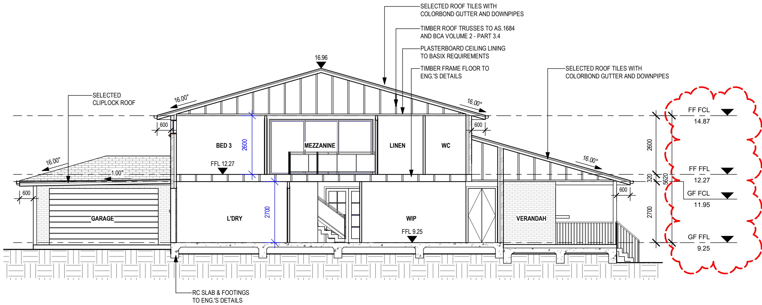
1 SECTION A-A 1 : 100
