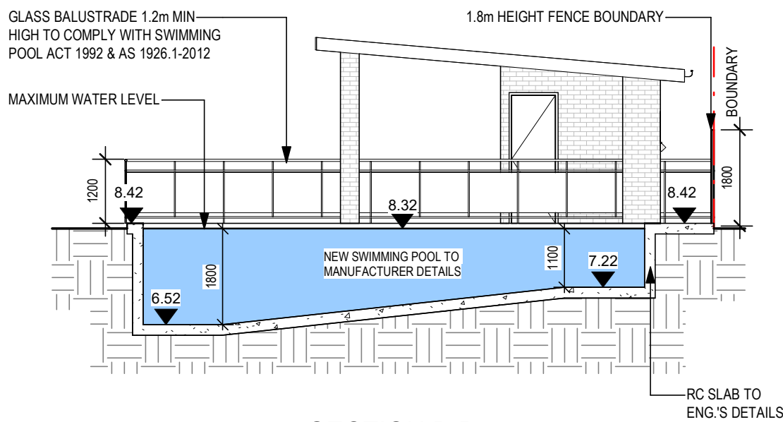
6 SECTION B-B 1 : 100
