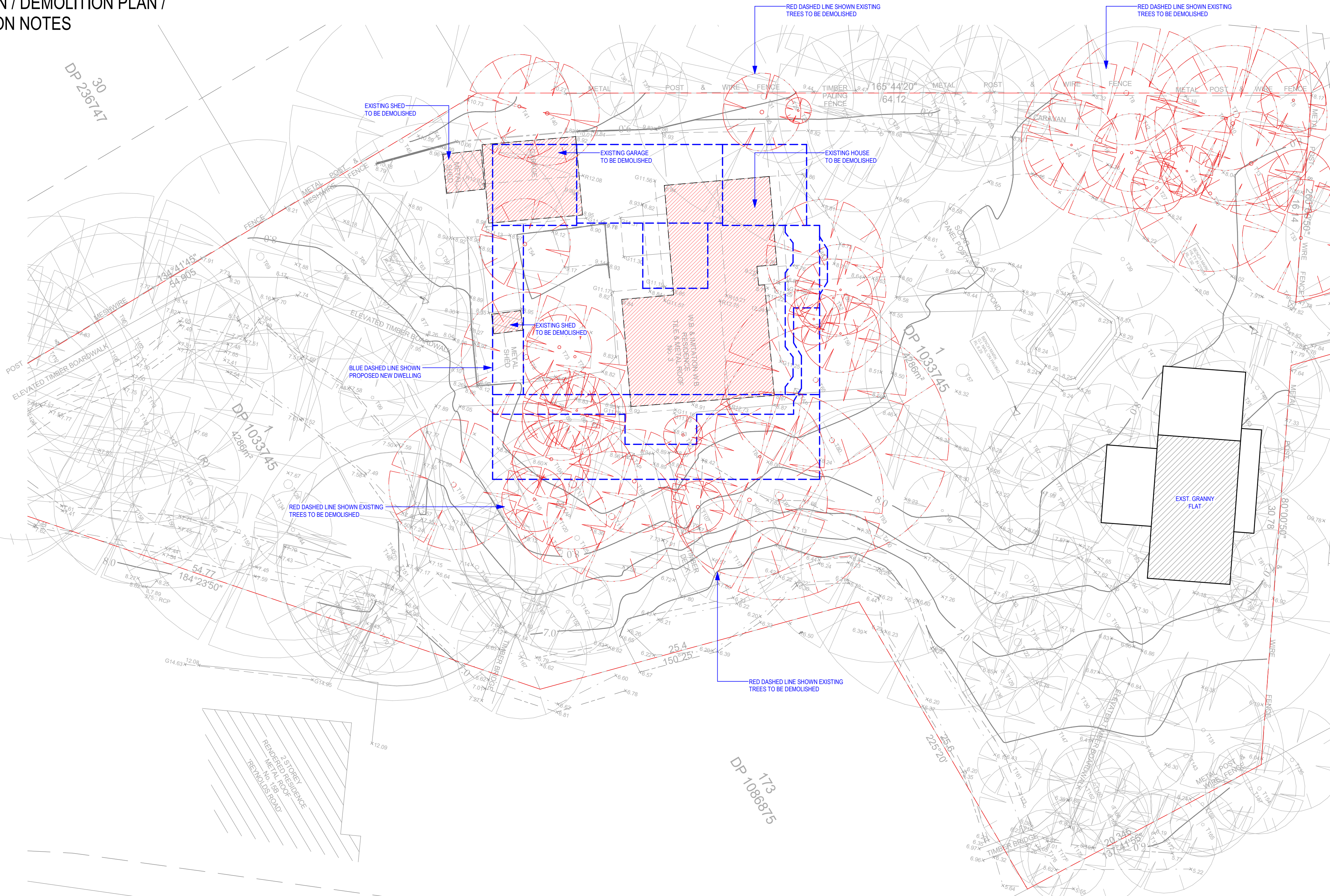
1 DEMOLITION PLAN 1 : 200
