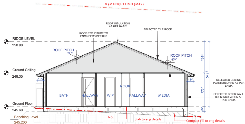
1 CROSS SECTION 1 : 100
