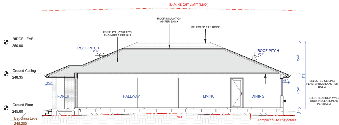
2 LONGITUDINAL SECTION 1 : 100
