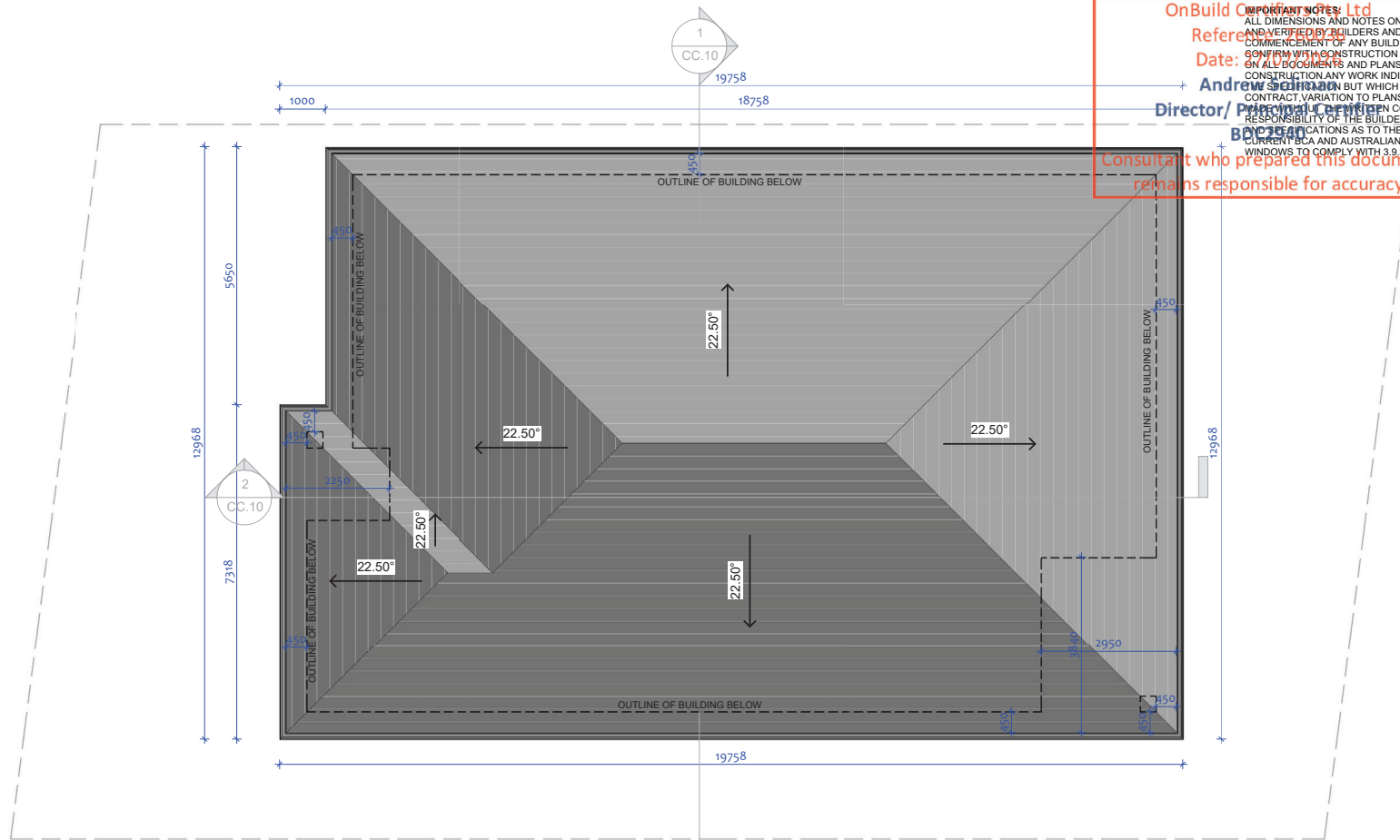
1 ROOF PLAN 1 : 100
