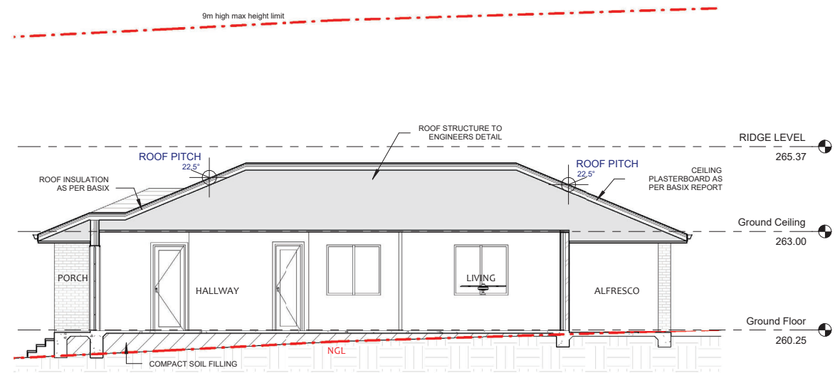
1 LONGITUDINAL SECTION 1 : 100
