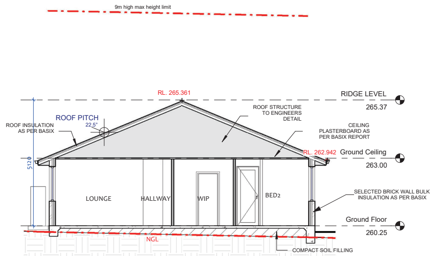
2 CROSS SECTION 1 : 100
