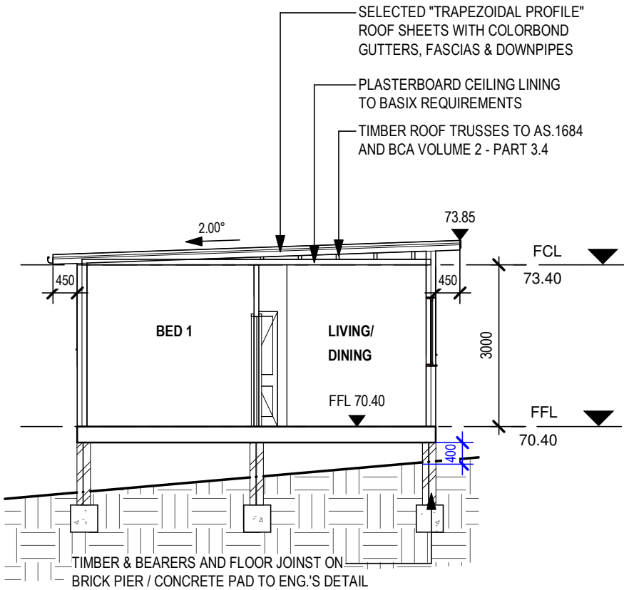
1 SECTION A-A 1 : 100
