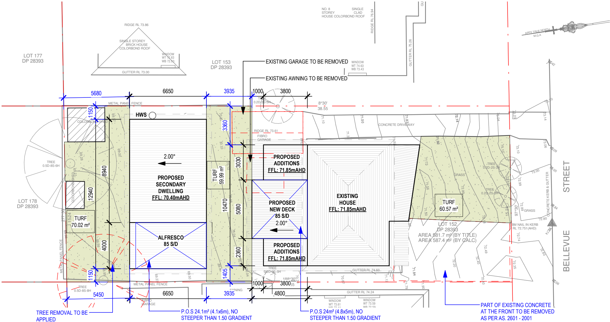
1 SITE & ROOF PLAN 1 : 200
