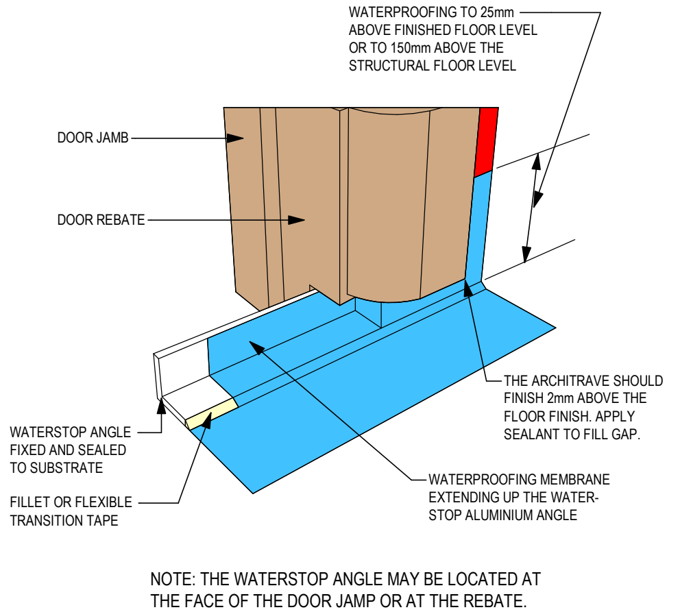
C05 WATERPROOFING UNDER DOOR ARCHITRAVE
