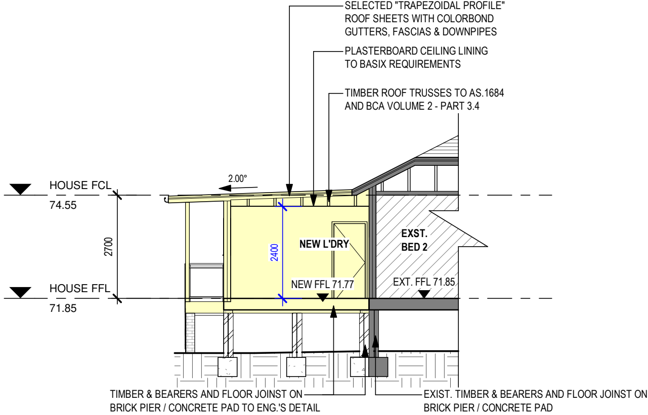
2 SECTION B-B 1 : 100
