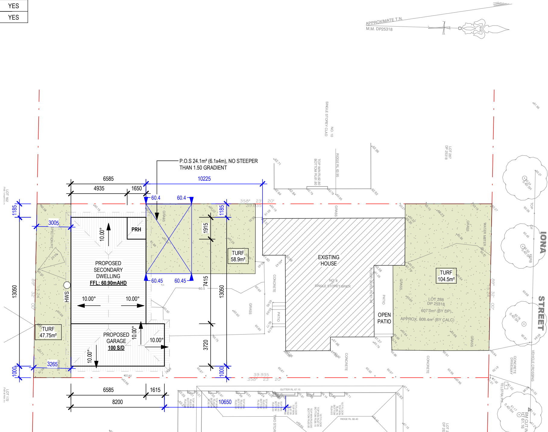
1 SITE & ROOF PLAN 1 : 200
