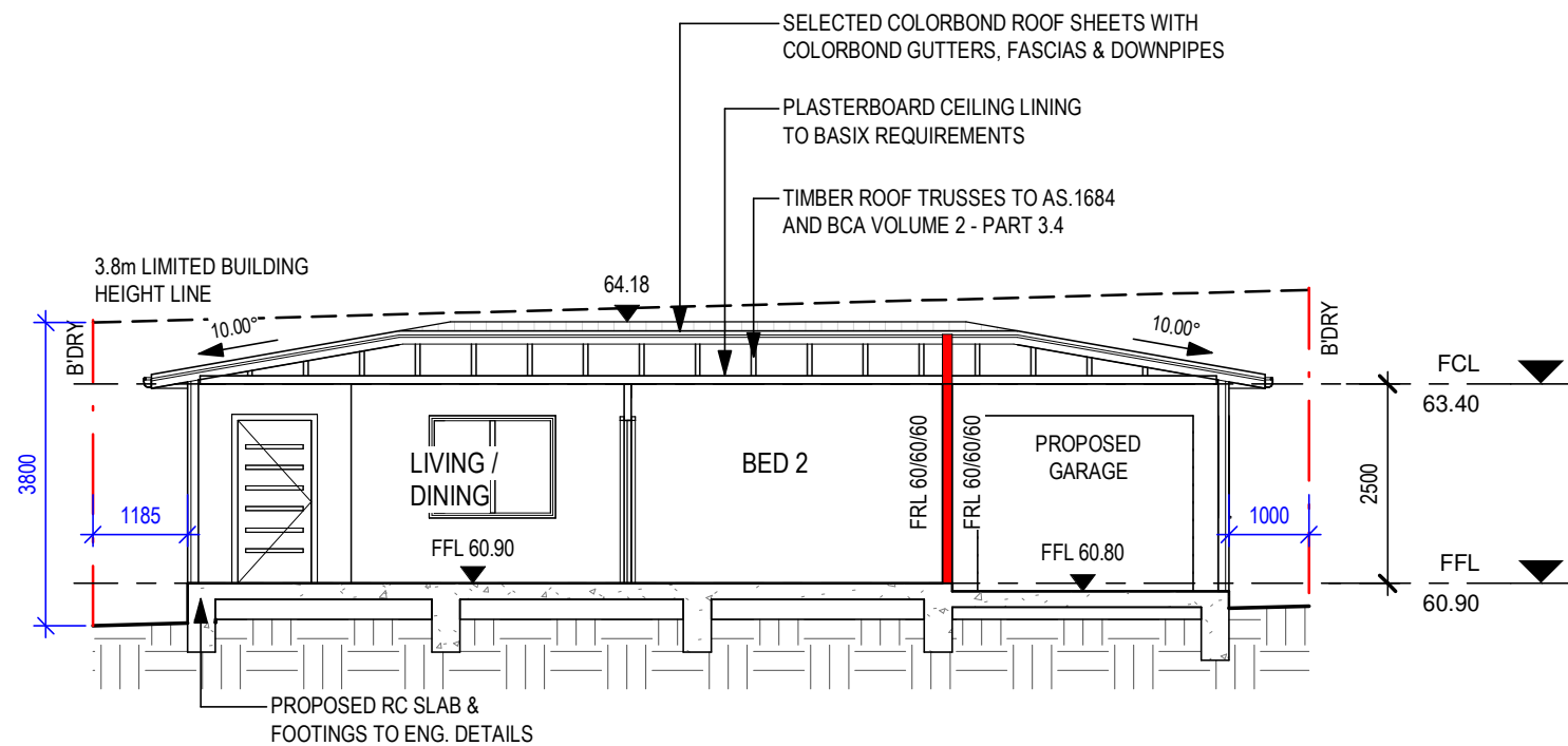
1 SECTION A-A 1 : 100
