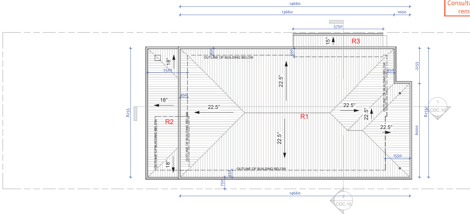
1 ROOF PLAN 1 : 100
