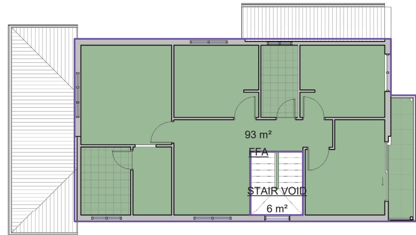
2 Level 1 1 : 100
