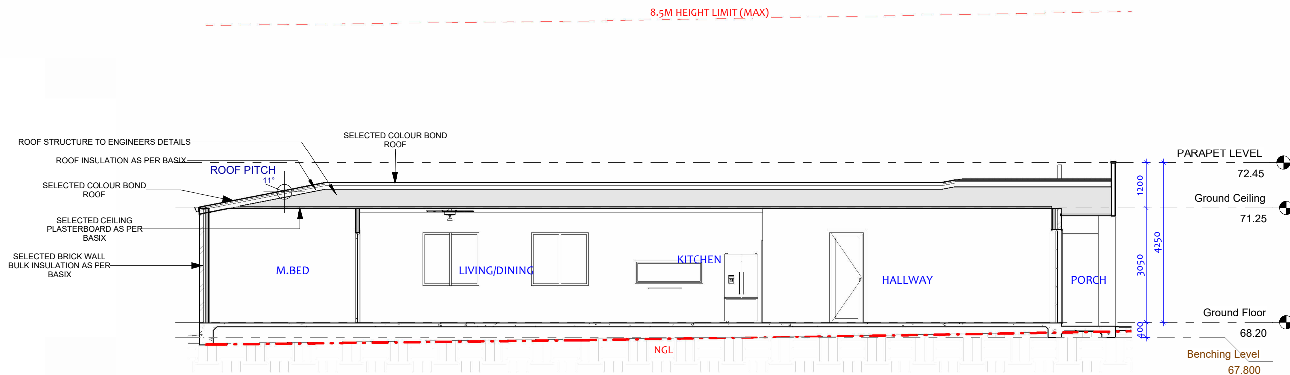
LONGITUDINAL SECTION 2 1 : 100
