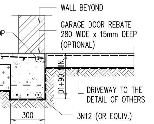
GARAGE EDGE BEAM – 'EB3'
