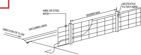
SEDIMENT FENCE - N.T.S
