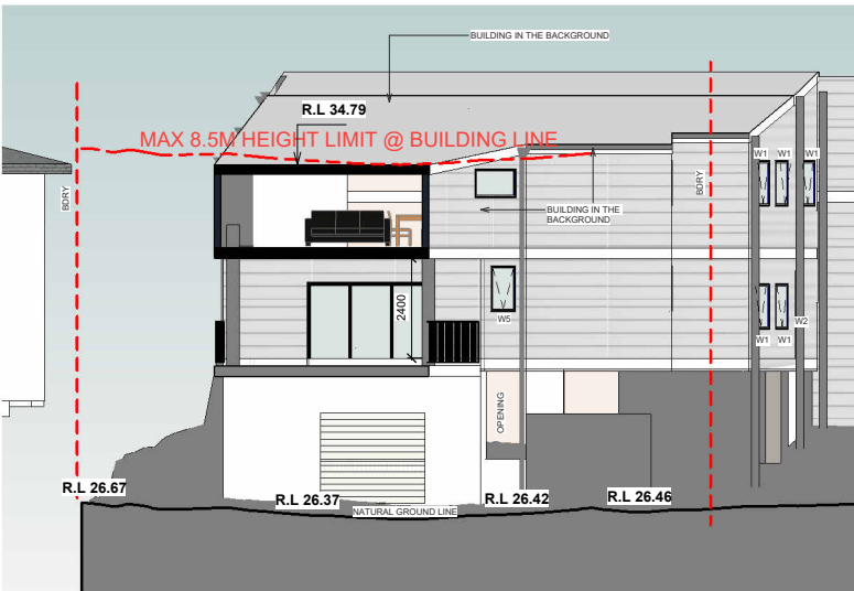
5 SECTION CC A008 1 : 100
