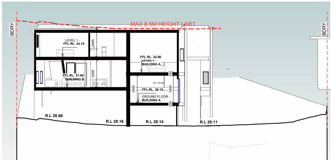
4 SECTION BB A008 1 : 100
