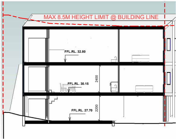
7 SECTION DD A008 1 : 100
