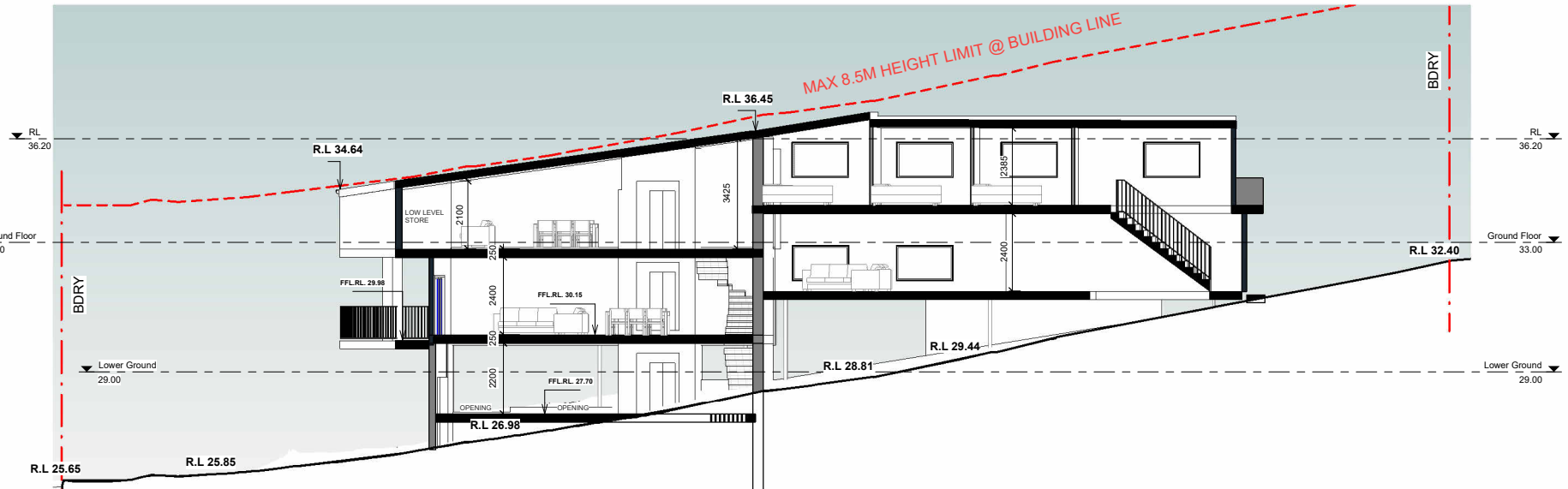
6 SECTION AA1 A008 1 : 100
