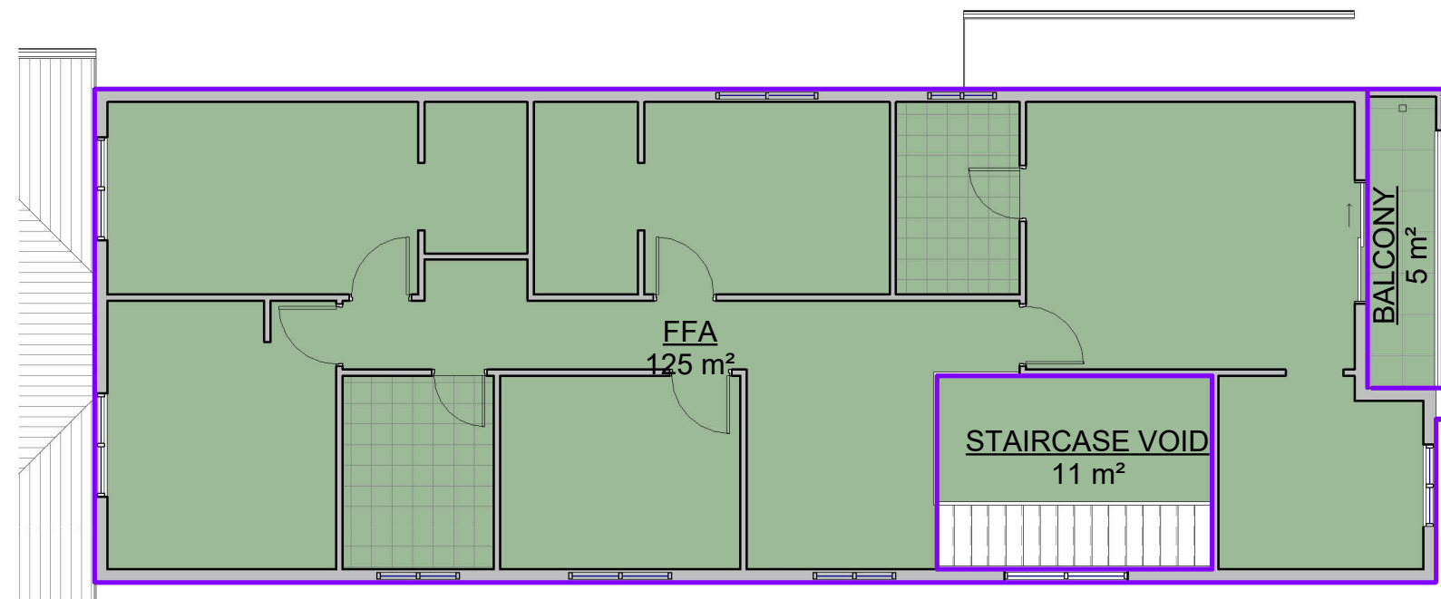
2 Level 1 1 : 100
