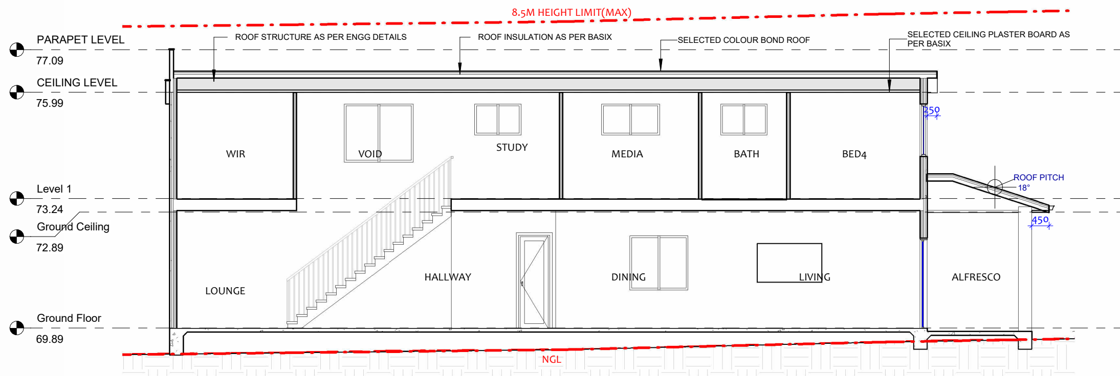
2 LONGITUDINAL SECTION 1 : 100
