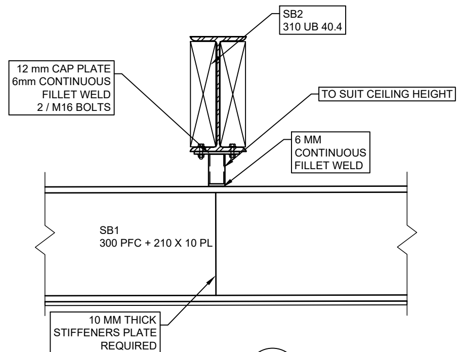
SECTION 2 scale 1 : 10
