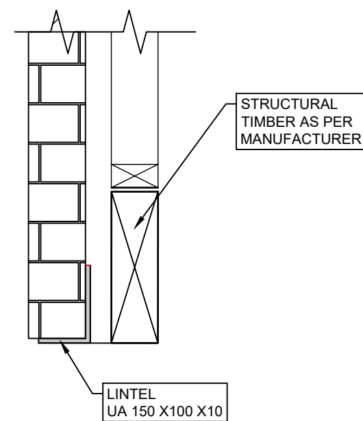
SECTION 4 scale 1 : 10
