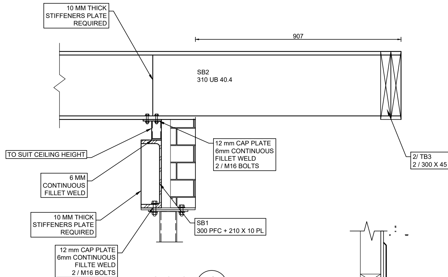
SECTION 1 scale 1 : 10
