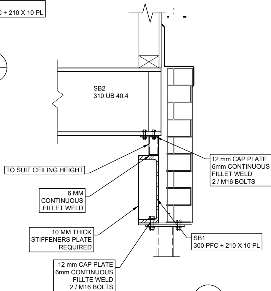
SECTION 3 scale 1 : 10
