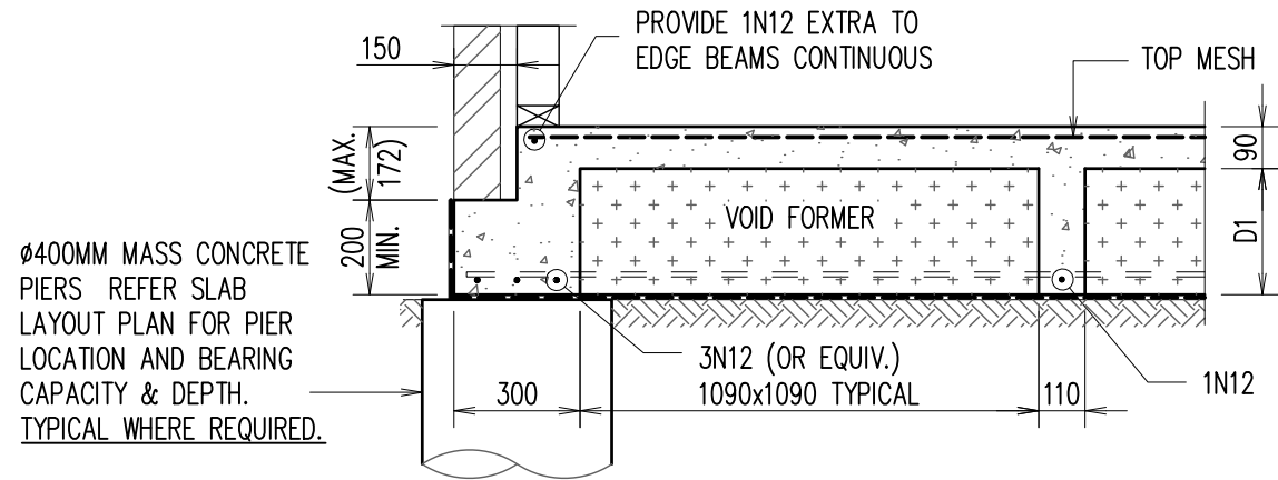
TYPICAL EDGE BEAM - 'EB1'
