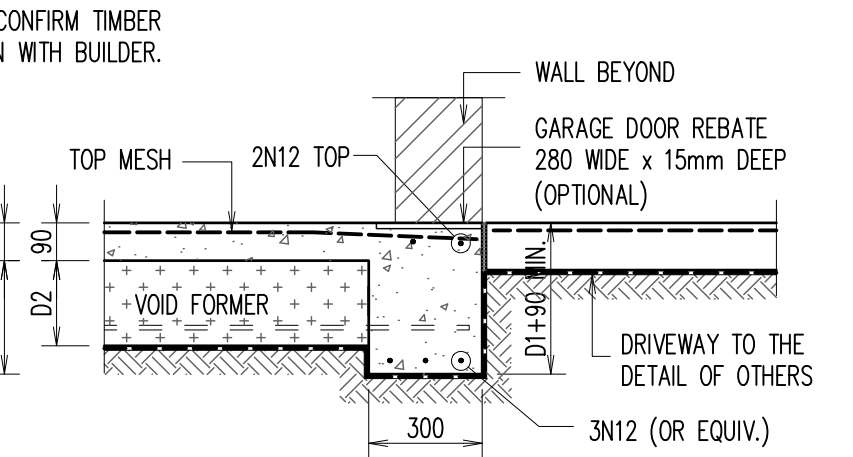
GARAGE EDGE BEAM - 'EB3'
