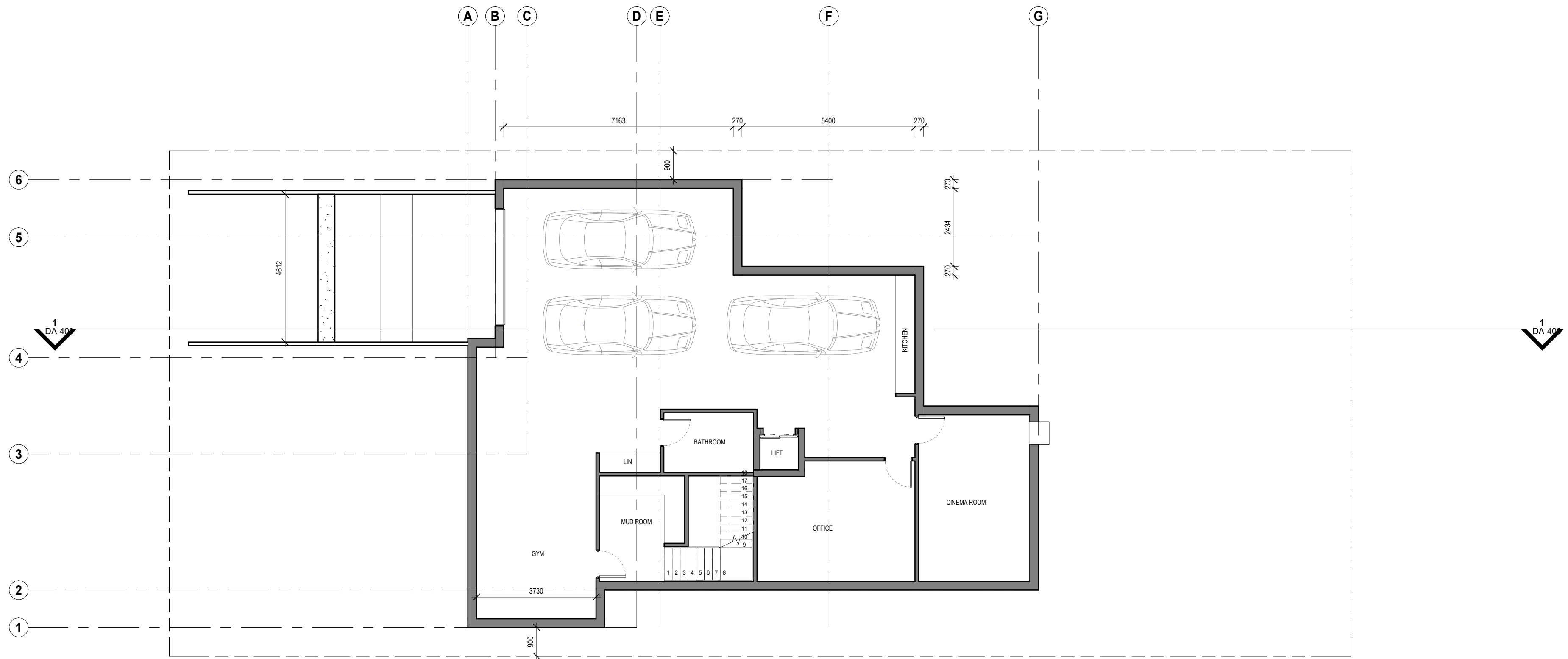
1 01 BASEMENT 1 : 100
