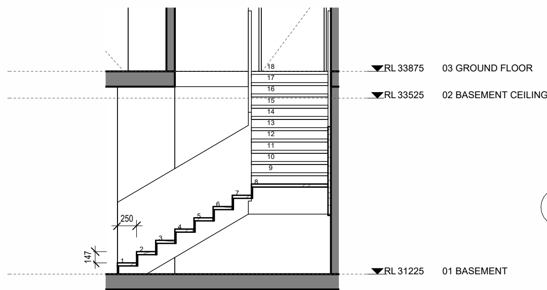
4 BASEMENT STAIR SECTION 1 : 50
