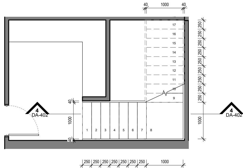
3 BASEMENT STAIRS 1 : 50
