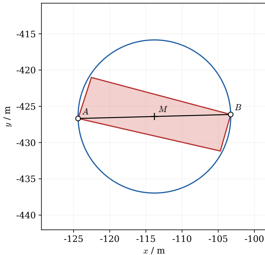
算例 A4：直径 21.1168 m；直径圆覆盖定位区域
