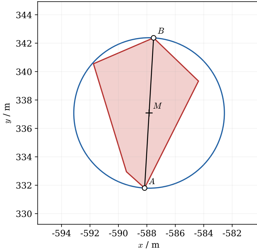
算例 A5：直径 10.5912 m；直径圆覆盖定位区域
