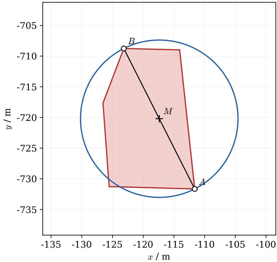
算例 A3：直径 25.6424 m；直径圆未覆盖定位区域
