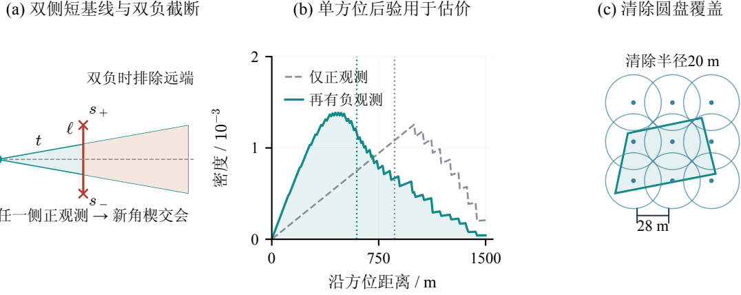
(a) 误差角示意放大10倍；实际 \eta \approx 1.005^\circ 。(b) 负测点为(550,180) m，竖线为均值。 后验均值不缩小保守可行域；清除覆盖依靠清除半径，不依赖信号接收方向。
