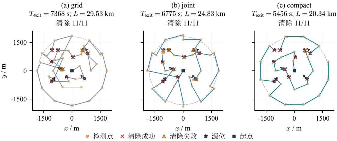
同一预定场景：源位及箭头均为退出后真值，箭头表示可接收半平面的中心方向。
