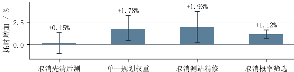
(b) 配对20局消融：均值及95%区间
