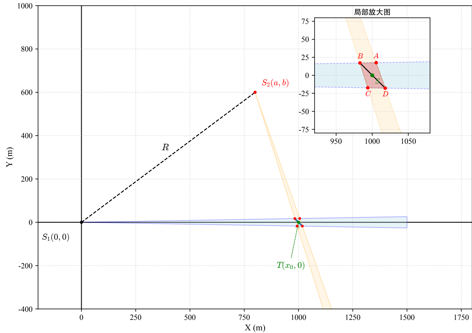
双测点示向度楔形交会几何分析示意图
