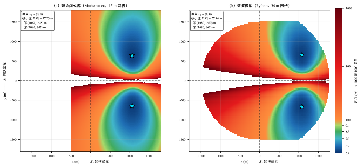
图 5 期望定位区域直径的分布：理论闭式解与数值模拟的并排对比。(a) Mathematica 按解析式在 15 \text{ m} 网格上求积；(b) Python 按交会四边形严格几何在 30 \text{ m} 网格上求解。两图的极小值位置与色带走向一致
