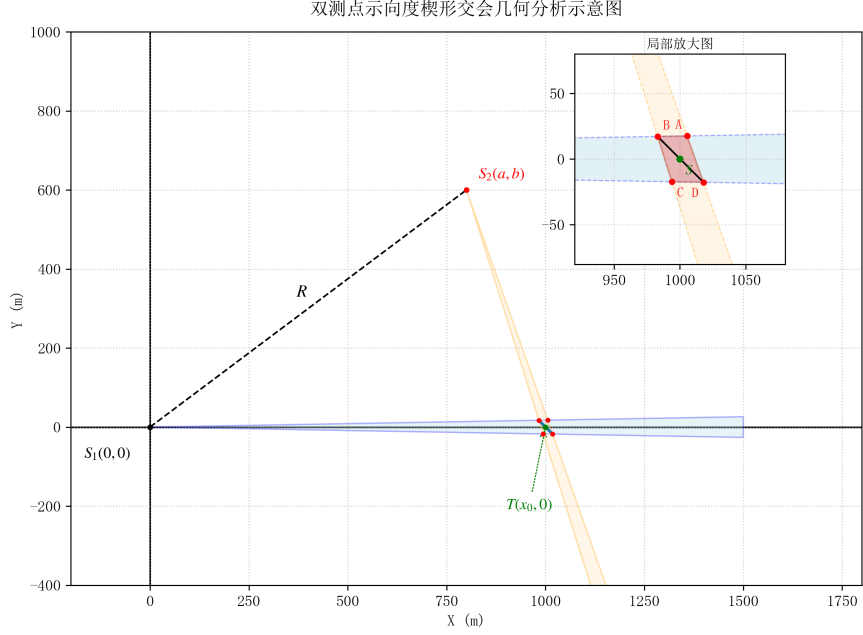
图 4 两探测束交会产生定位区域示意图
