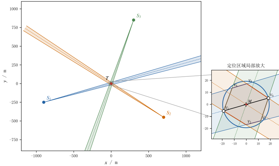
图 1 多检测点示向度交会定位；右侧局部图保留各色角楔边界，并标出交点 V_i 和直径中点 M
