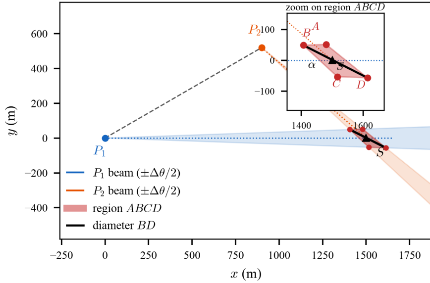
图 3 两探测束交会与探测域直径的构造（半张角放大 2 倍示意）
