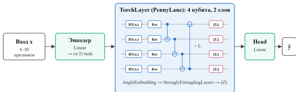
Рисунок 1 – Гибридная модель Hybrid QNN на основе PennyLane
