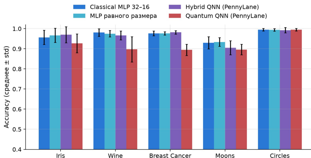
Рисунок 3 – Ассигуру классических моделей и моделей PennyLane (среднее \pm стандартное отклонение)
