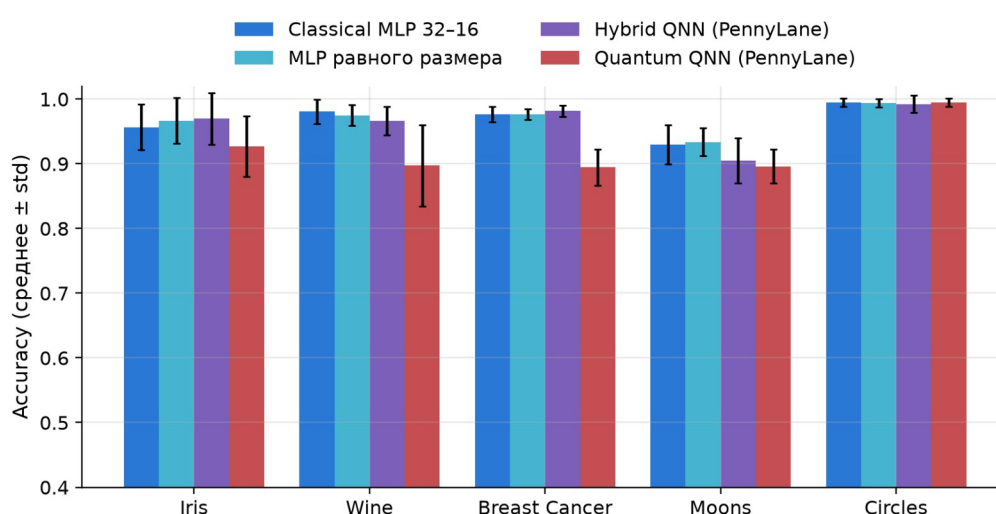
Рисунок 3 – Аксурасу классических моделей и моделей PennyLane (среднее ± стандартное отклонение)
