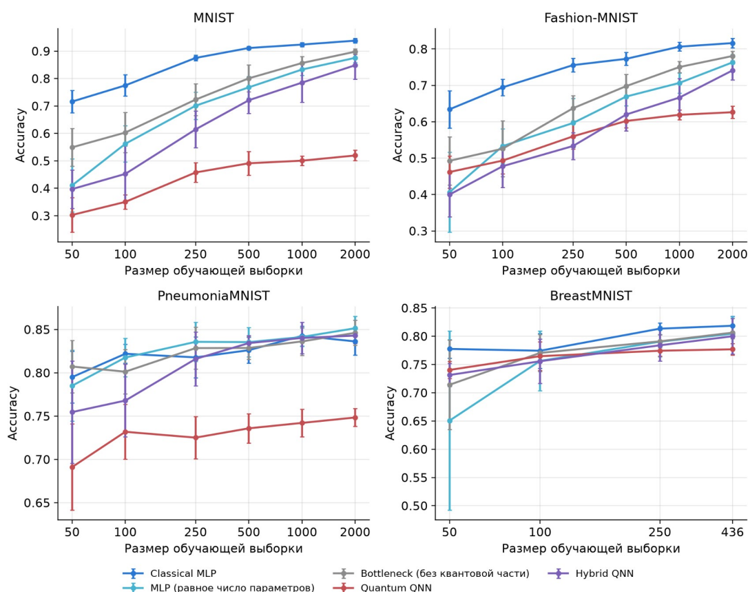
Рисунок 7 – Ассигасу моделей на изображениях в зависимости от размера обучающей выборки (4 кубита)
