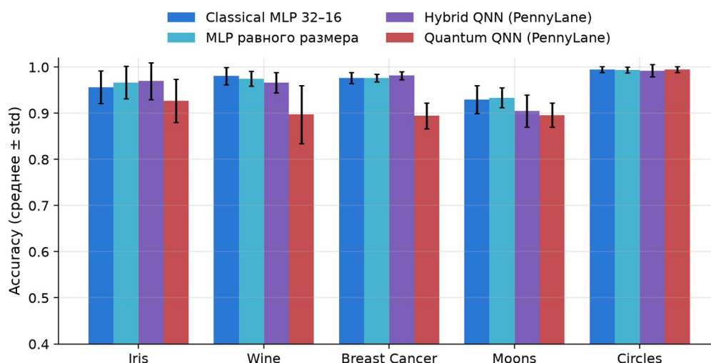
Рисунок 3 – Accuracy классических моделей и моделей PennyLane (среднее \pm стандартное отклонение)
