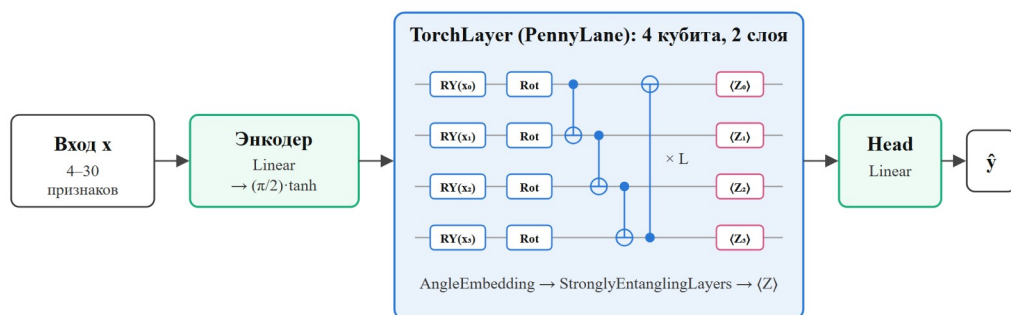
Рисунок 1 – Гибридная модель Hybrid QNN на основе PennyLane
