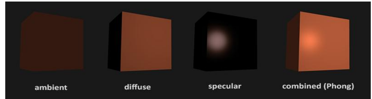
Компоненты модели Фонга
