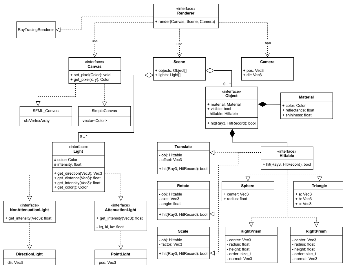
Рисунок 3.1 – Диаграмма классов приложения
