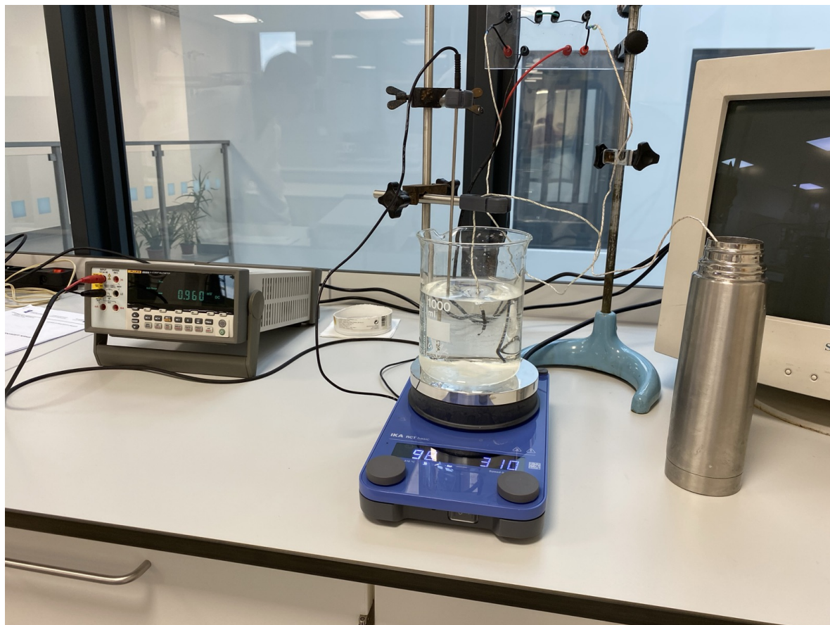
Rysunek 1: Zdjęcie stanowiska pomiarowego dla części dotyczącej wyznaczania charakterystyki kalibracyjnej termopary
