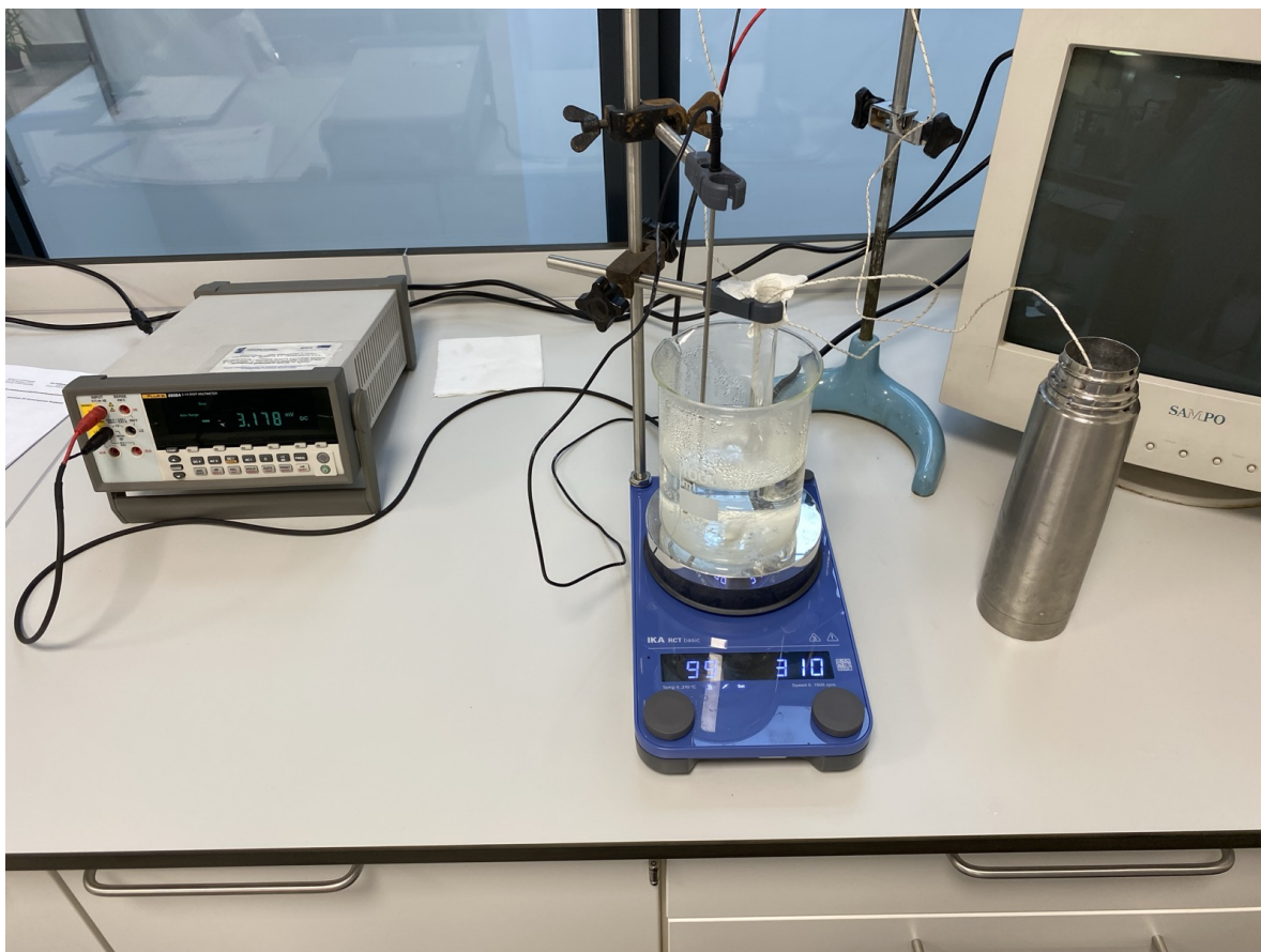
Rysunek 2: Stanowisko pomiarowe do określenia temperatury przemiany fazowej stopu
