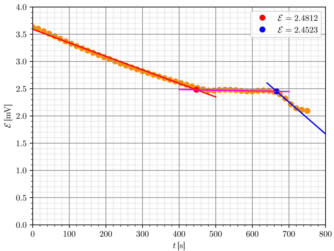
Rysunek 5: Chłodzenie
