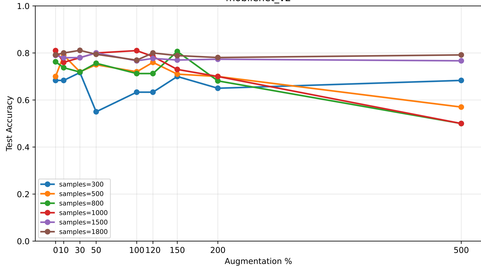
mobilenet_v2
